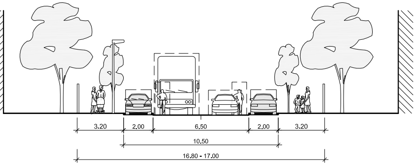
Querschnitt A-A geplanter Querschnitt
