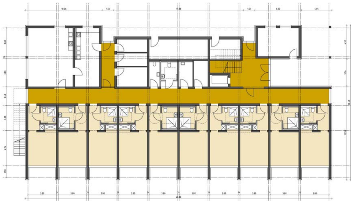
Grundriss Pflege
