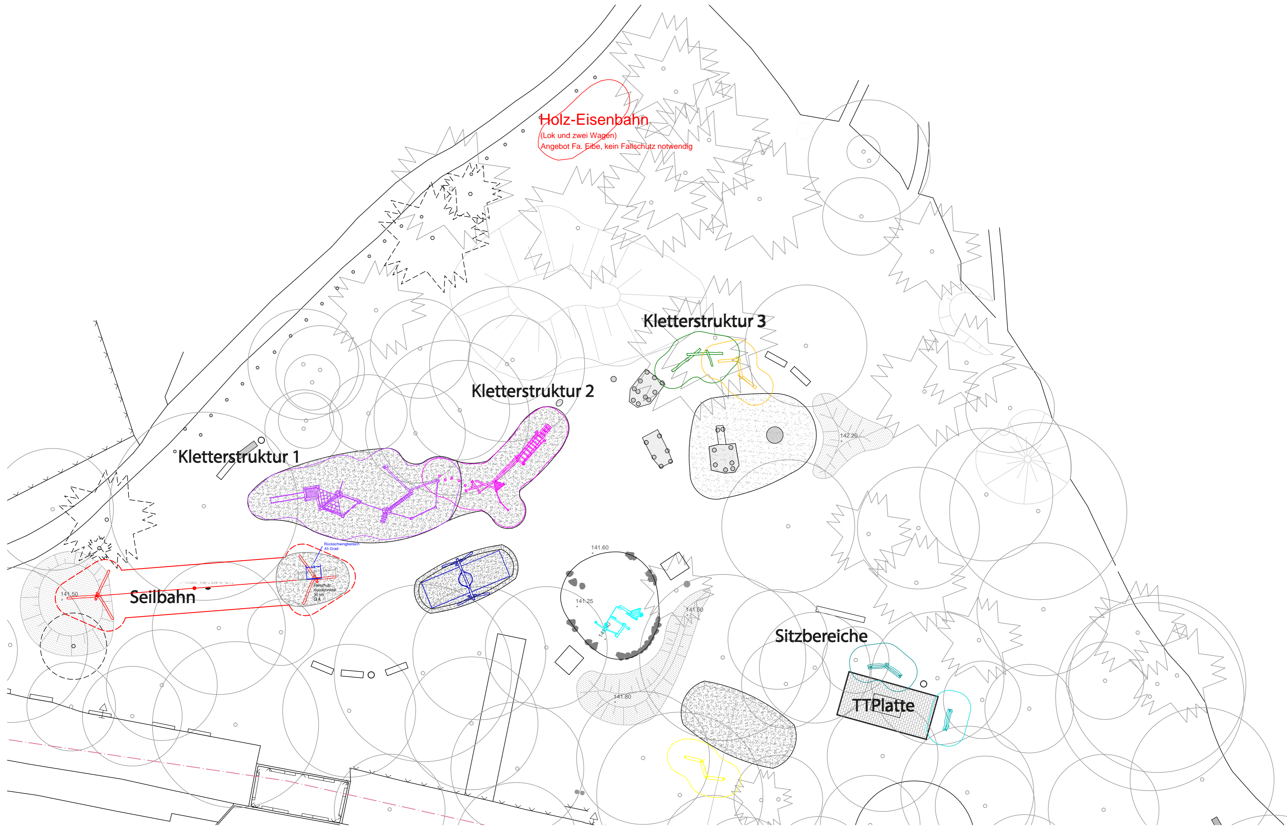
Sanierung Spielplatz Neuländer Straße Dresden - Lageplan mit Einordnung Eisenbahn M 1:200, Stand: 31.10.2020
