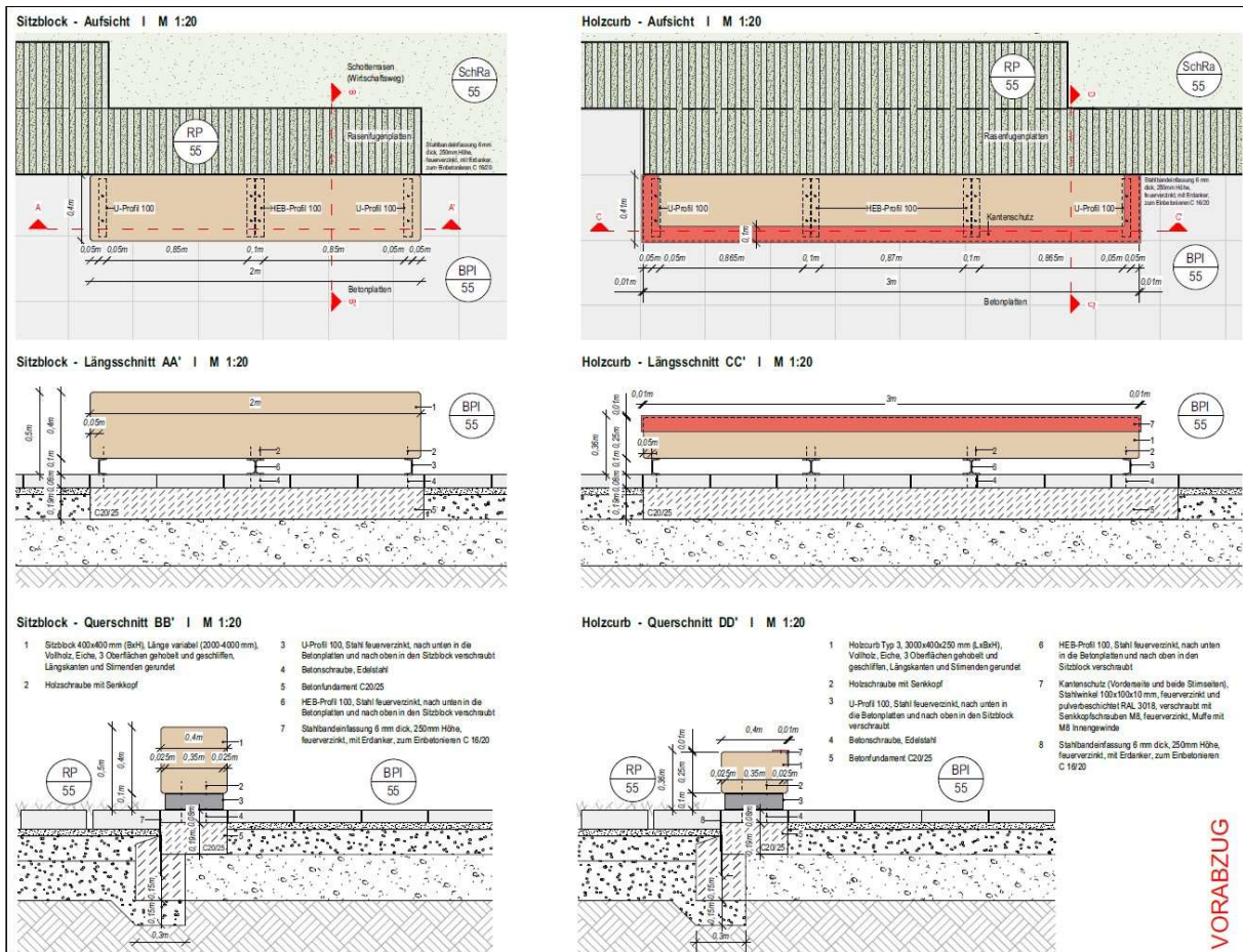
Detail Sitzblöcke und Holzcurbs (QuerFeldEins Dresden, ohne Maßstab)
